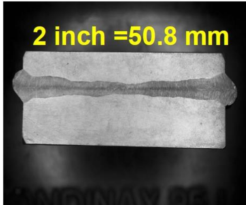
2 吋 (50.8 mm) 雙面焊接 20kW 不鏽鋼 1.4301
